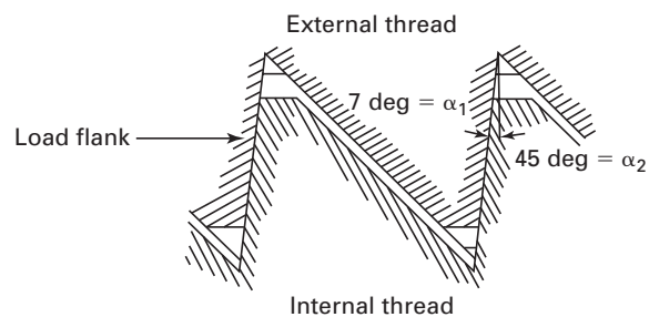
Fig. 31 Load Flank
