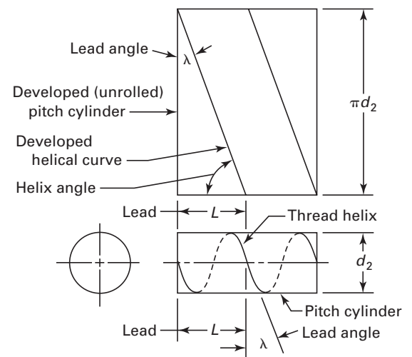
Fig. 21 Helix
